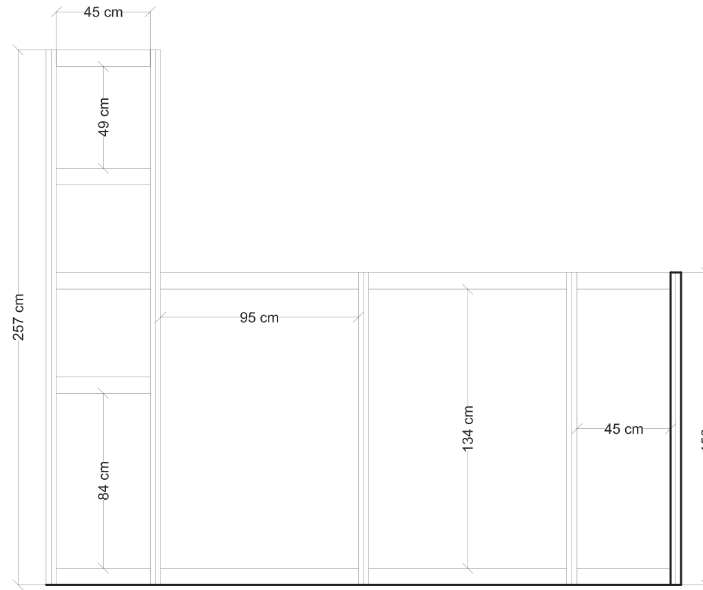
ALZADO
