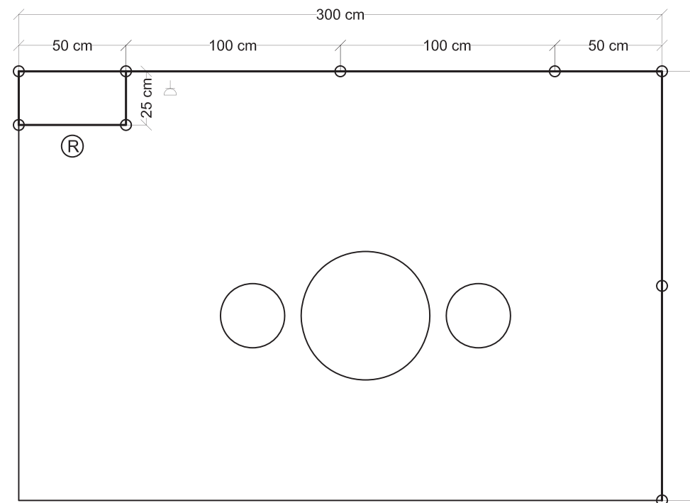
PLANTA
